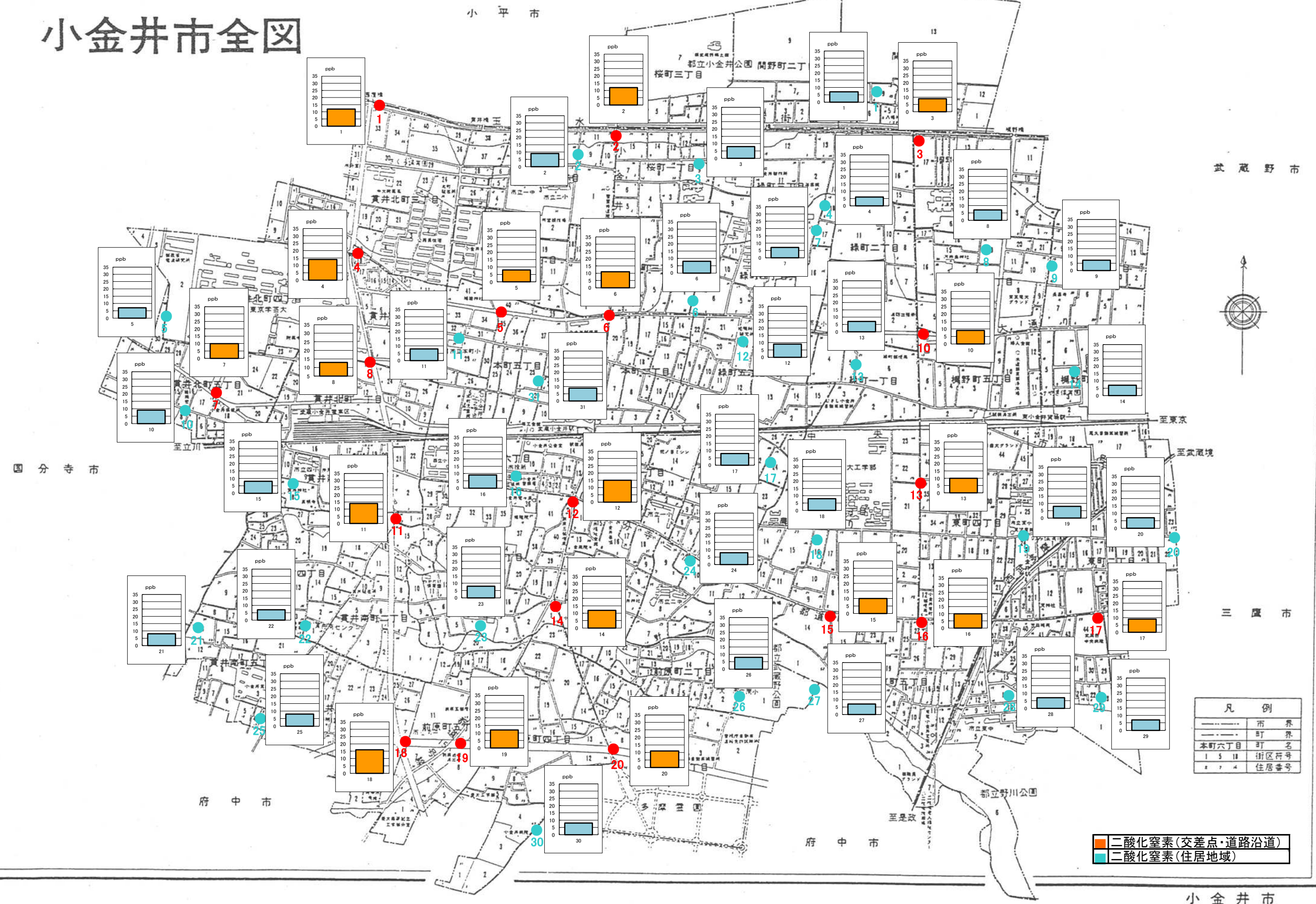
図 2 二酸化窒素調査結果図(令和7年度)
