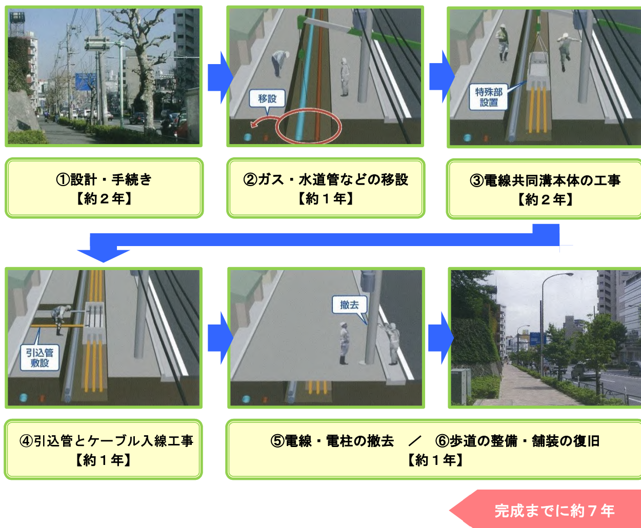
図 2.12 電線共同溝方式による無電柱化の整備手順と整備期間
