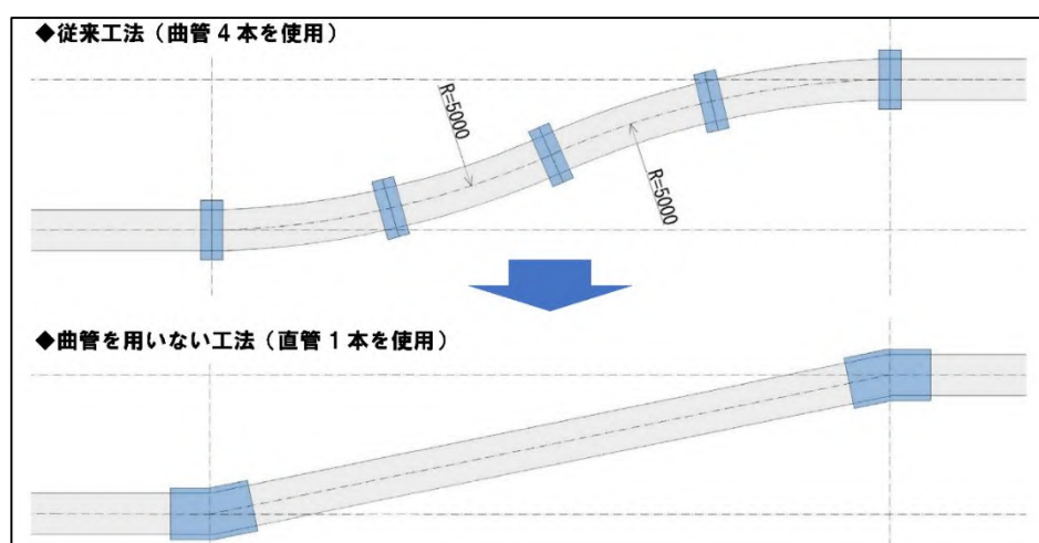
図 5.3 曲管を用いない工法（イメージ）
