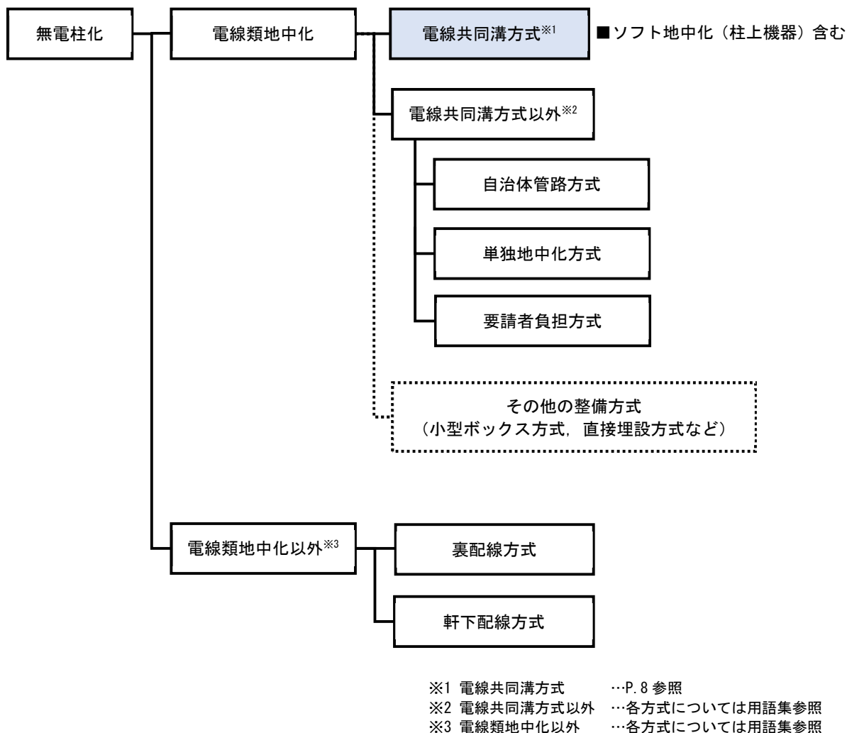
図 2.3 無電柱化の整備方式と整備手法
