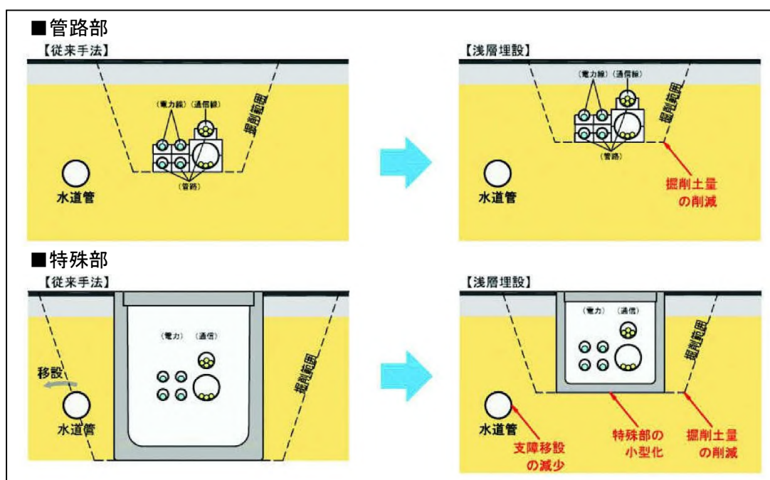
図 5.4 浅層埋設による低コスト化（イメージ）
