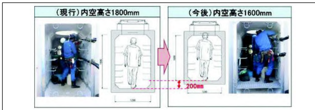
図 5.2 特殊部のコンパクト化による低コスト化（イメージ）
