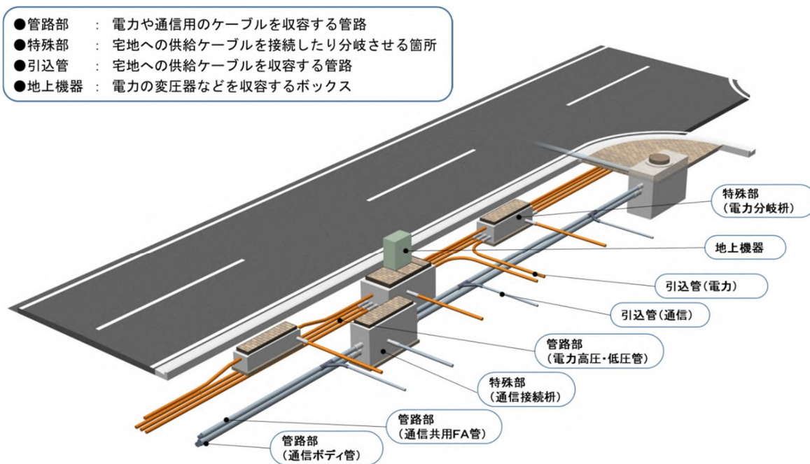
図 2.4 道路区域内に地上機器を設置する電線共同溝のイメージ
