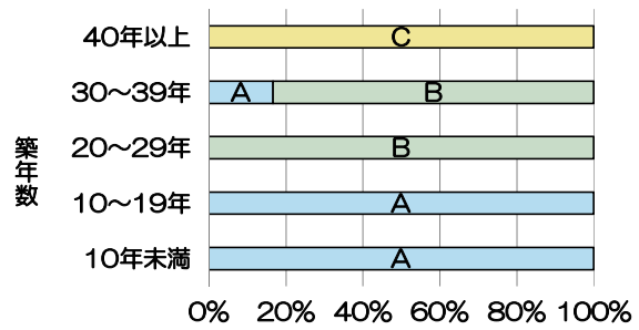
図10 機械設備の築年数別劣化状況
