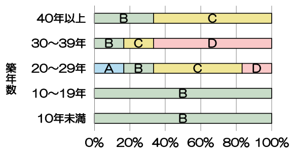
図 7 外壁の築年数別劣化状況
