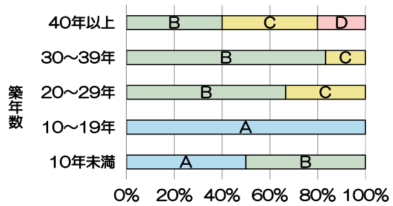
図8 内部仕上の築年数別劣化状況
